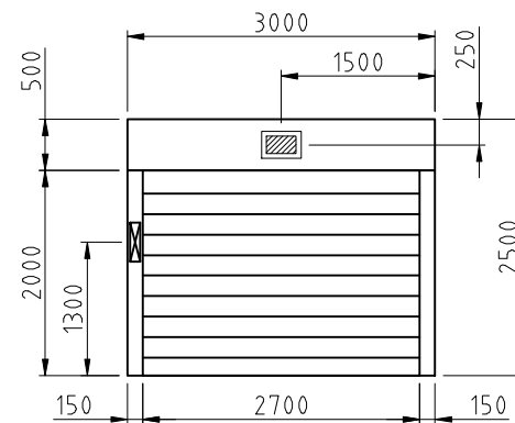
出入口詳圖
