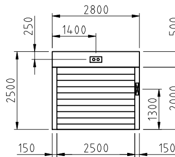
BF 出入口詳圖
