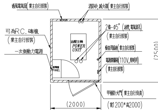
機械房標準平面圖 *機械室詳細位置經業主確認後告知
