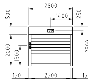
1F 出入口詳圖
