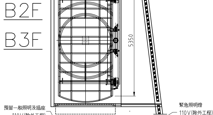
出入口詳圖 #多餘之間隙，請業主於門板安裝完成後予以修飾(除外工程)
