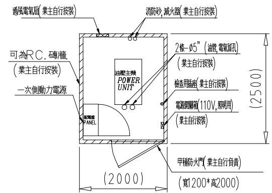
機械房標準平面圖
