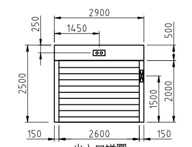
出入口詳圖
