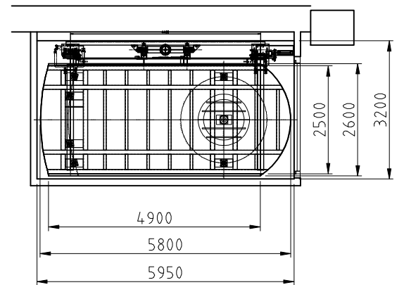
1F 昇降道平面圖
